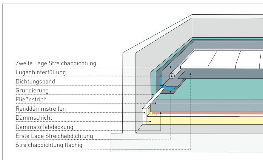
Streichabdichtung
